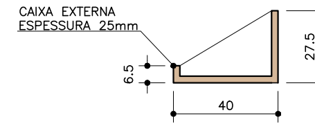
EXPOSITOR VINIL . CORTE CAIXA EXTERNA ESC. 1:20
