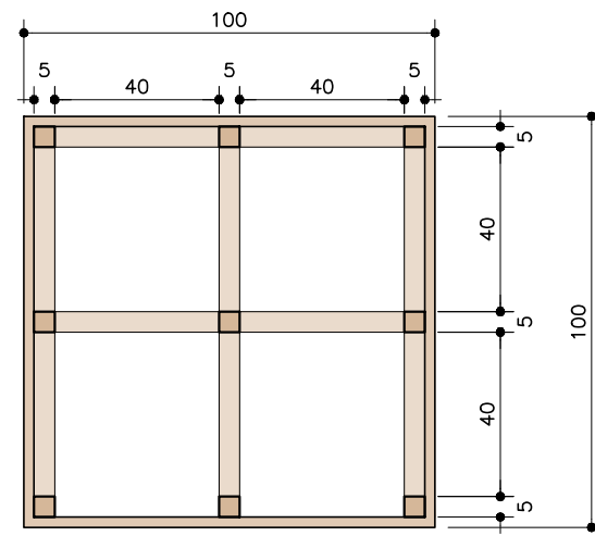
MÓDULO PRATICAVÉL . PLANTA INFERIOR ESC. 1:20
