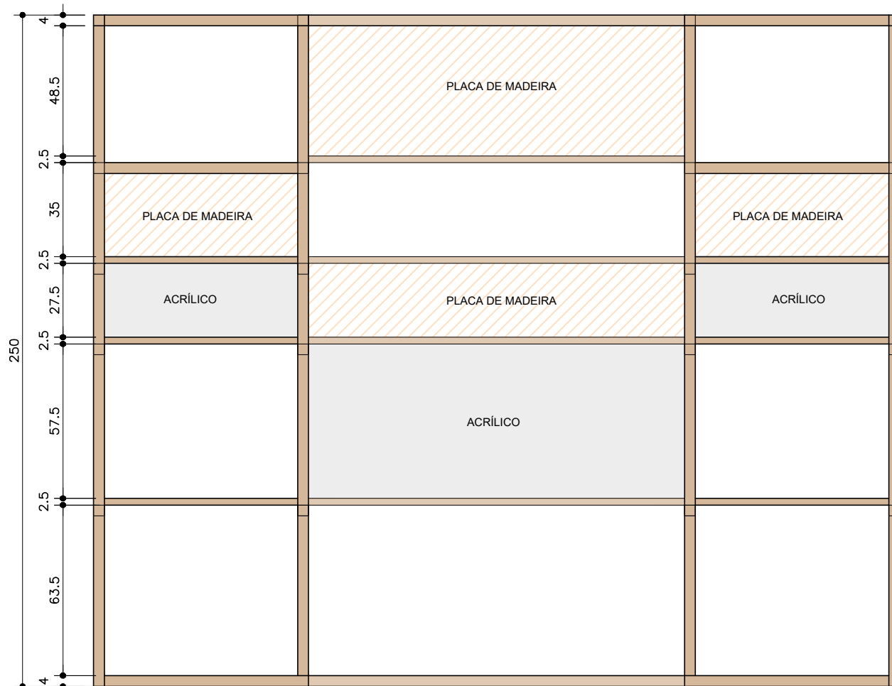
ESTANTE . VISTA FRONTAL ESC. 1:20
