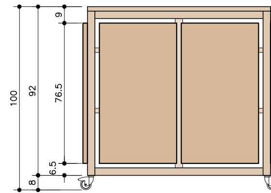
BALCÃO RECEPÇÃO . VISTA FRONTAL ESC. 1:20
