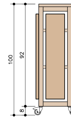
BALCÃO RECEPÇÃO . VISTA LATERAL ESC. 1:20
