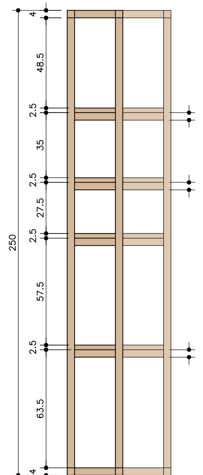
ESTANTE . VISTA LATERAL ESC. 1:20
