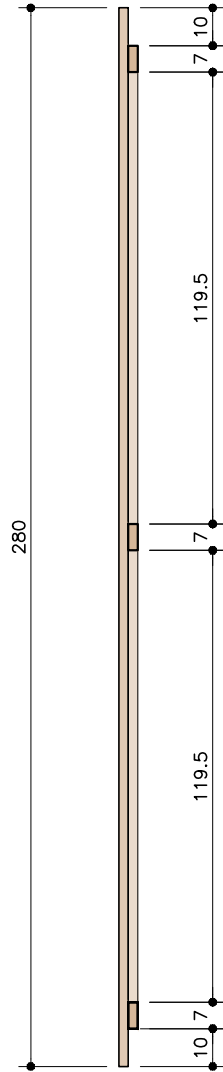
PLACA SALA EXPOSIÇÃO . VISTA LATERAL ESC. 1:20
