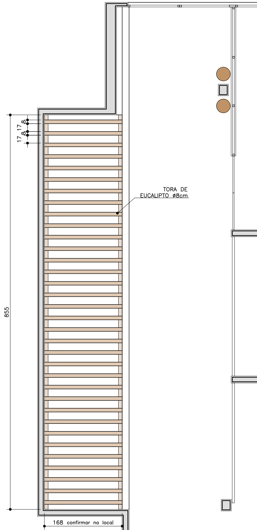
PLANTA . PERGOLADO ESC. 1:50
