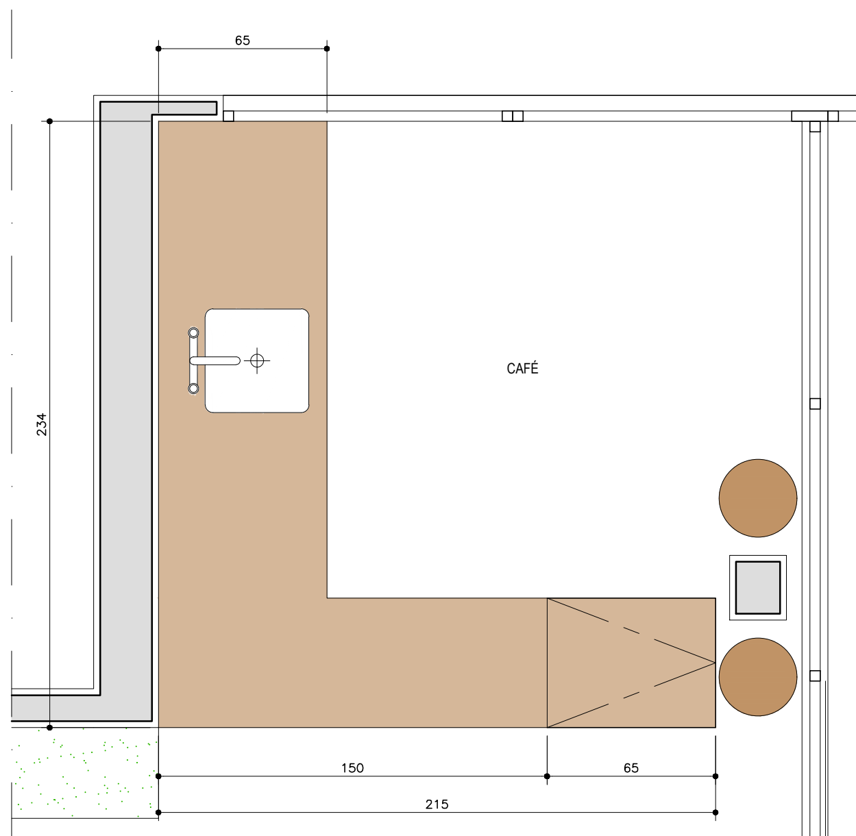
CAFÉ . PLANTA LAYOUT ESC. 1:20
