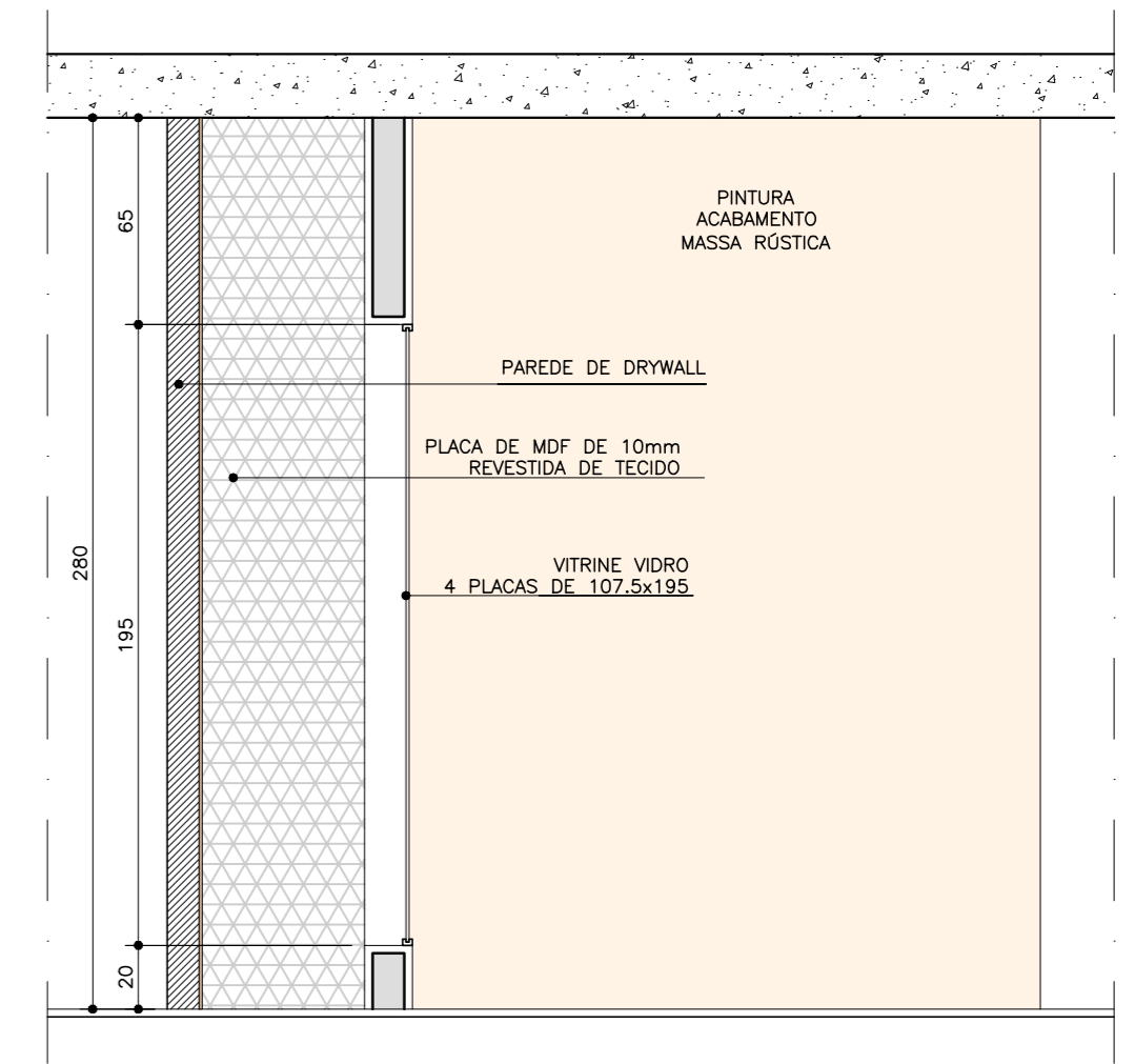
PAREDE DRYWALL . CORTE AA ESC. 1:25
