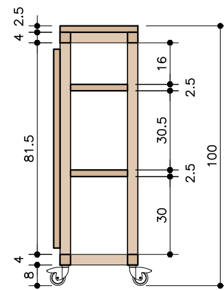
BALCÃO RECEPÇÃO . CORTE TRANSVERSAL ESC. 1:20
