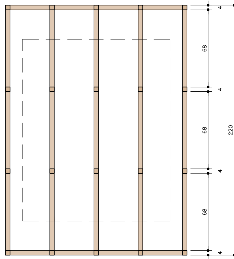
PAINEL EXPOSITOR . CORTE A ESC. 1:20
