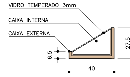
EXPOSITOR VINIL . CORTE TRANSVERSAL ESC. 1:20
