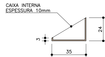
EXPOSITOR VINIL . CORTE CAIXA INTERNA ESC. 1:20
