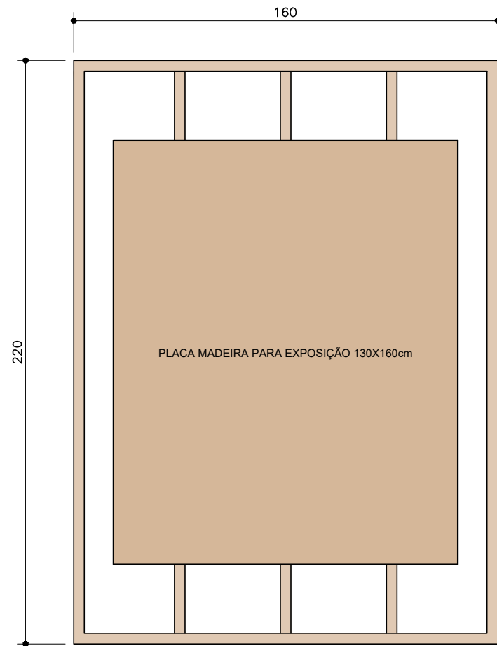
PAINEL EXPOSITOR . VISTA FRONTAL ESC. 1:20
