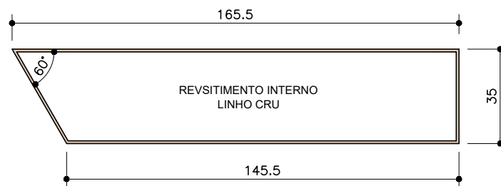
EXPOSITOR VINIL . PLANTA CAIXAS INTERNAS ESC. 1:20
