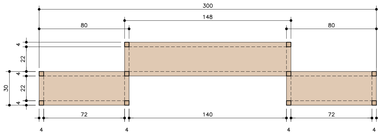
ESTANTE . PLANTA ESC. 1:20
