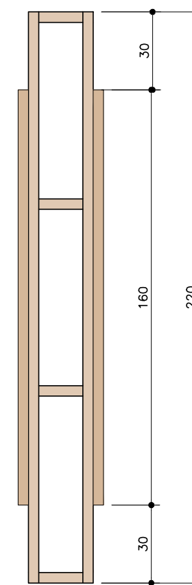
PAINEL EXPOSITOR . VISTA LATERAL ESC. 1:20
