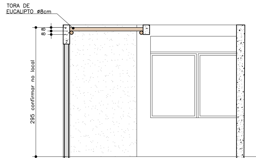
CORTE . PERGOLADO ESC. 1:50
