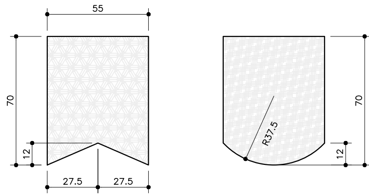
ESTANDARTES . VISTA FRONTAL
