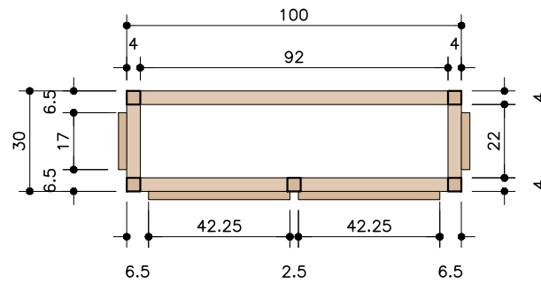
BALCÃO RECEPÇÃO . PLANTA ESC. 1:20
