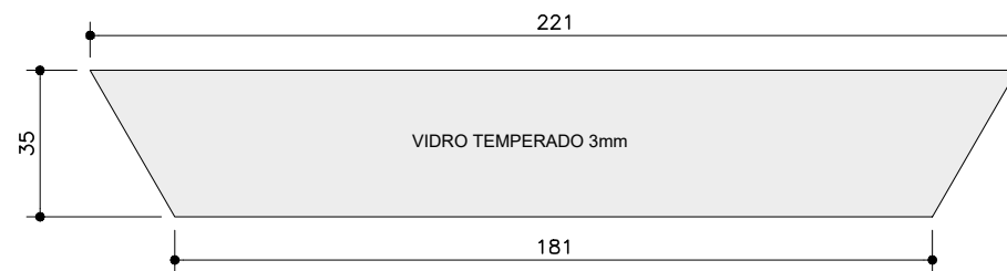
VIDRO EXPOSITOR VINIL . PLANTA ESC. 1:20
