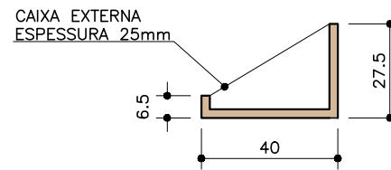
EXPOSITOR VINIL . CORTE CAIXA EXTERNA ESC. 1:20
