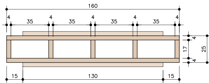
PAINEL EXPOSITOR . PLANTA ESC. 1:20
