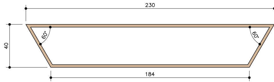
EXPOSITOR VINIL . PLANTA CAIXA EXTERNA ESC. 1:20
