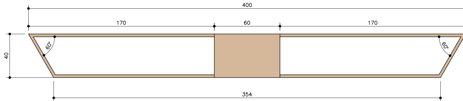
EXPOSITOR VINIL . PLANTA CAIXA EXTERNA ESC. 1:20
