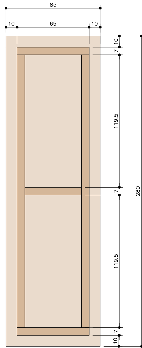
PLACA SALA EXPOSIÇÃO . VISTA TRASEIRA ESC. 1:20
