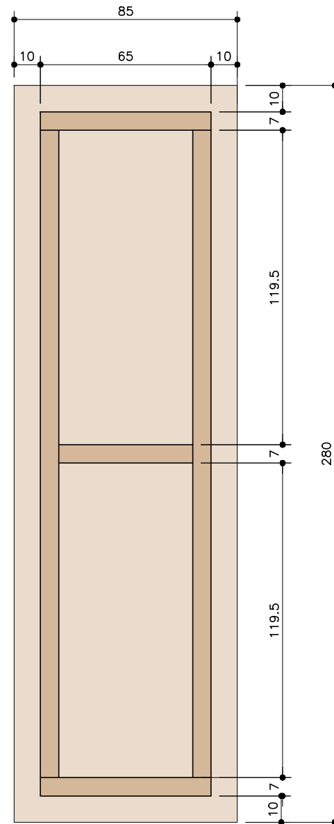
PLACA SALA EXPOSIÇÃO . VISTA TRASEIRA ESC. 1:20
