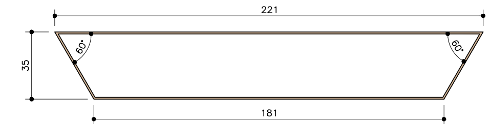
EXPOSITOR VINIL . PLANTA CAIXA INTERNA ESC. 1:20
