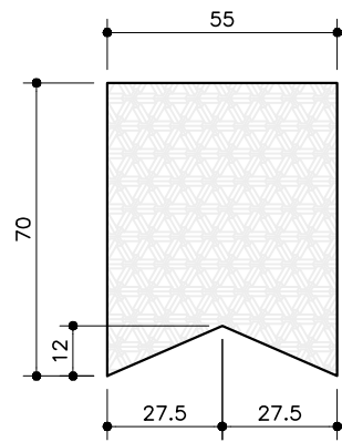
ESTANDARTES . VISTA FRONTAL
