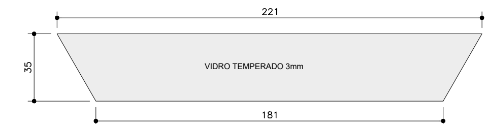
VIDRO EXPOSITOR VINIL . PLANTA ESC. 1:20
